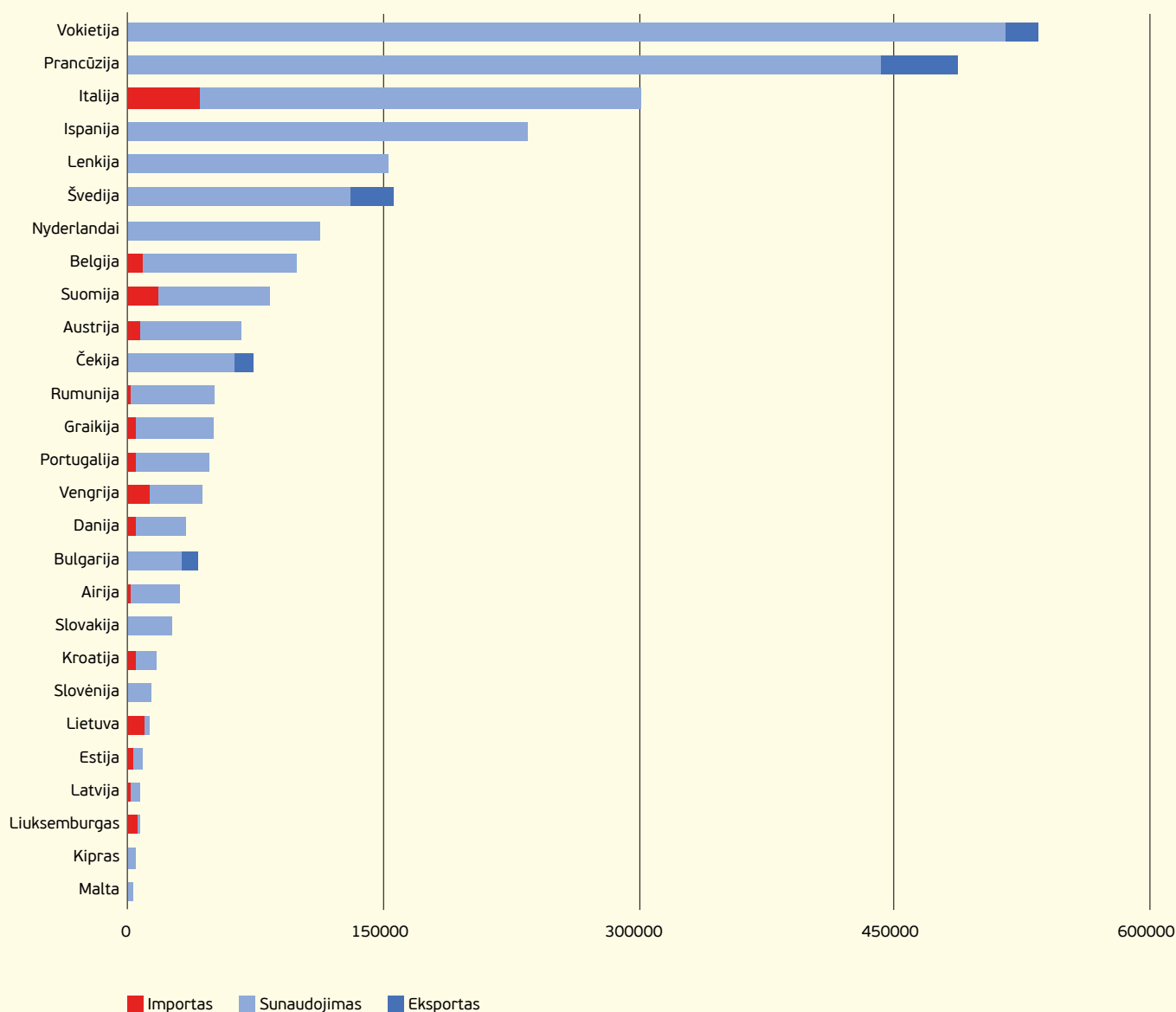
Elektros gamyba ir suvartojimas ES valstybėse, GWh
